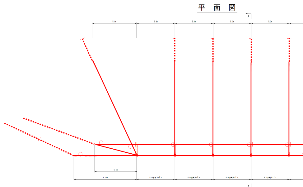
標準断面図
