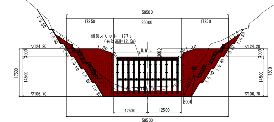
正面図
