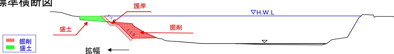
標準横断面図
