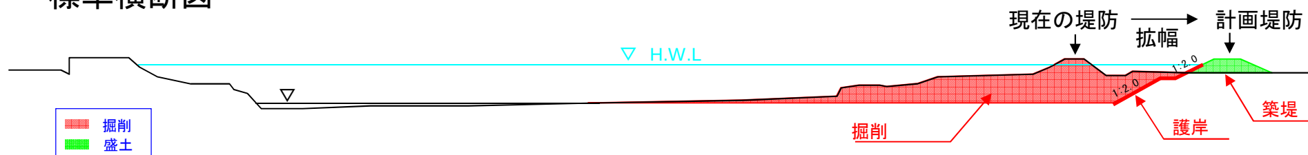
標準横断面図
