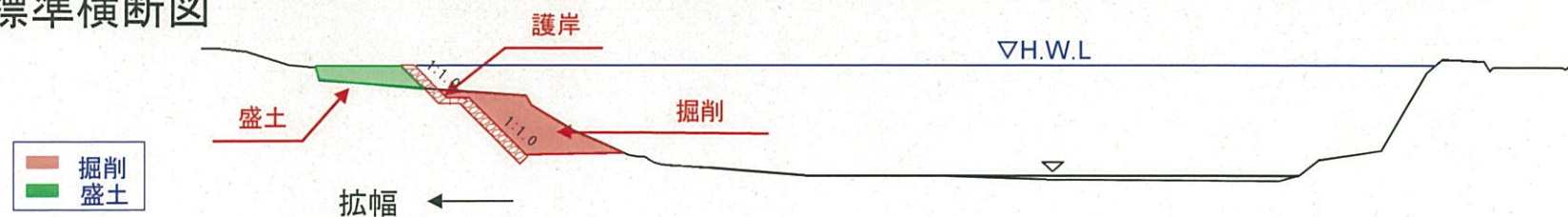
標準横断面図
