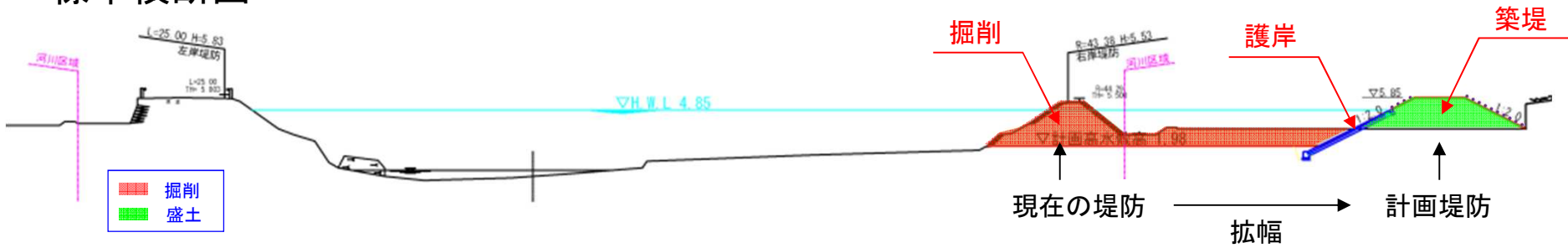
標準横断図
