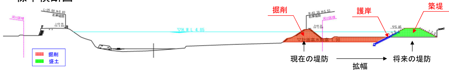
標準横断面図
