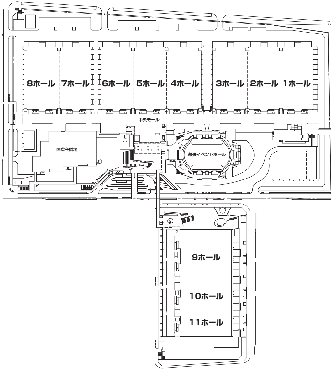
① 建設諸元 制限床荷重 最大 1~9ホール 5t/m 2 10・11ホール 3t/m 2
