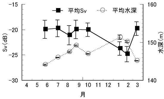
図2 海底面から海底面下10mまでの平均体積戻り散乱強度(海底面下平均 Sv)の経時変化(50m×20回の平均±標準偏差)
