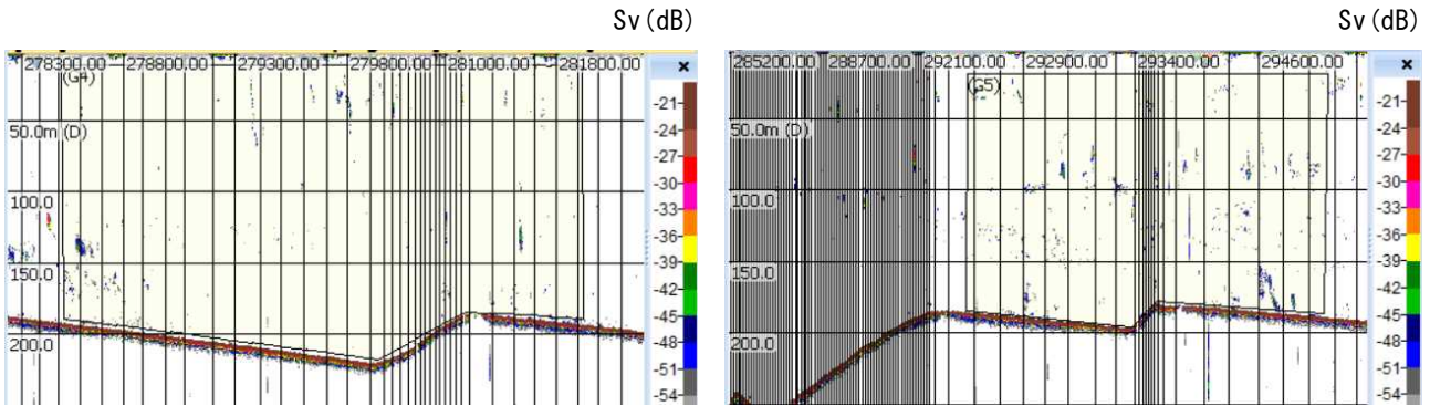
図3 2015年2月25日の釣獲調査時のエコーグラム(Sv)(グリッド, 縦(水深)50m×横100m) 左図, 解析グループG4; 右図, 解析グループG5(図1および表1参照)。
