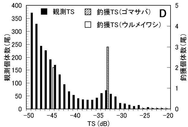
図4 魚探で観測されたTSと釣獲個体(主要浮魚類)から推定されたTSの関係 A, 2014年12月8日(G1); B, 2015年2月24日(G1-3); C, 2015年2月25日(G4); D, 2015年2月25日(G5)。解析グループ(G)は図1および表1参照。
