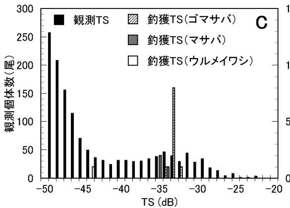
図4 魚探で観測されたTSと釣獲個体(主要浮魚類)から推定されたTSの関係 A, 2014年12月8日(G1); B, 2015年2月24日(G1-3); C, 2015年2月25日(G4); D, 2015年2月25日(G5)。解析グループ(G)は図1および表1参照。
