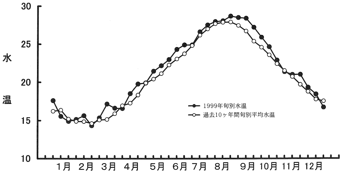
図2 1999年旬別水温と過去10ヶ年間（'89～'98）旬別平均水温
