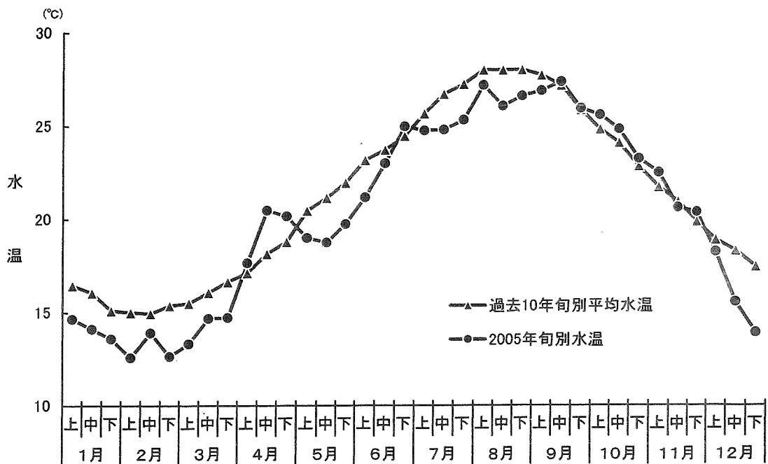
図2 2005年の旬別水温と過去(1995~'04年)の旬別平均水温
