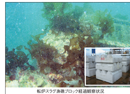
転炉スラグ漁礁ブロック経過観察状況
