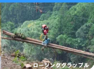
油圧式集材機
