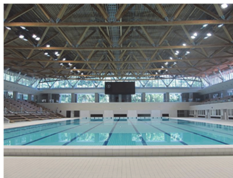
屋根の架構に使用されたスギ大断面のハイブリッド材（和歌山県秋葉山県民水泳場）
