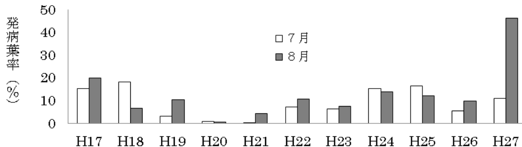
図2 モモせん孔細菌病の発病葉率(調査時期:7月、8月、調査園数10園)
