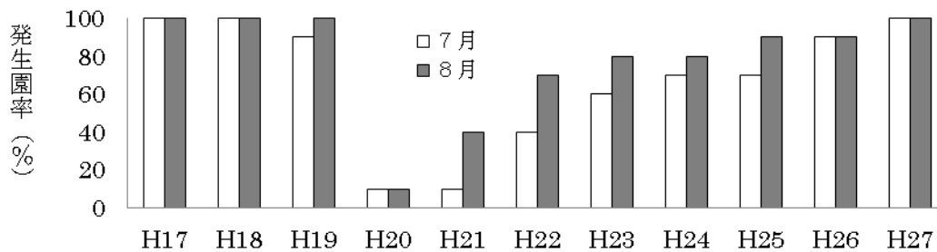
図1 モモせん孔細菌病の発生園率(調査時期:7月、8月、調査園数10園)
