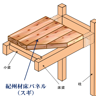
構造用床パネルの開発イメージ
