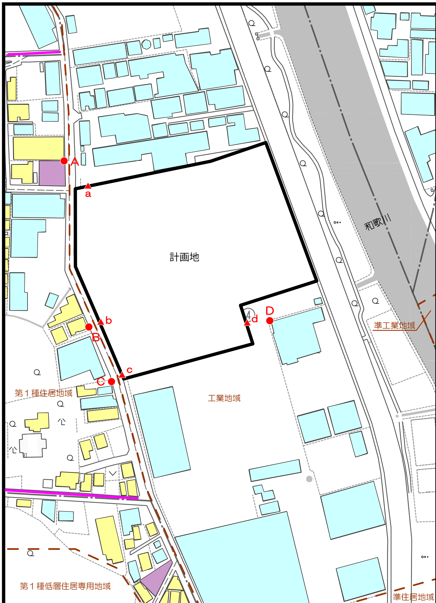
付図1 周辺見取図兼騒音予測地点図
