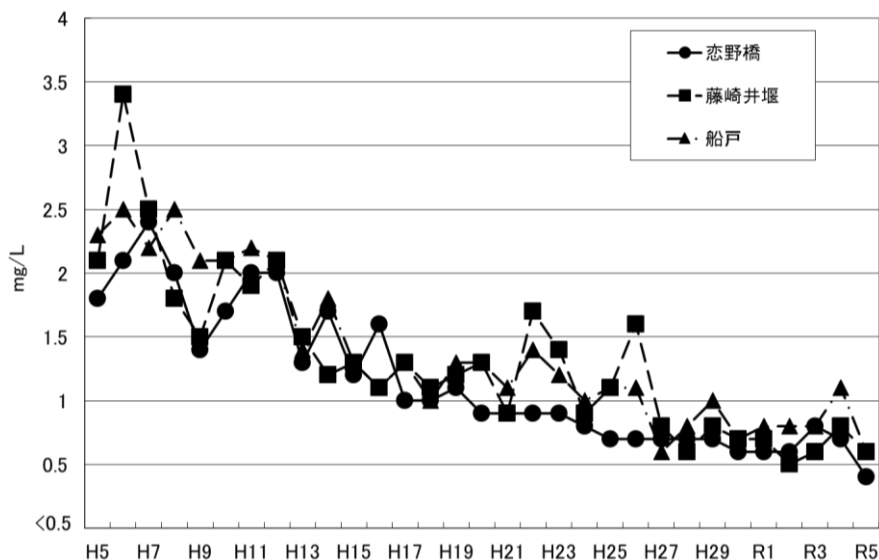
② 紀の川のBOD75%値の推移
