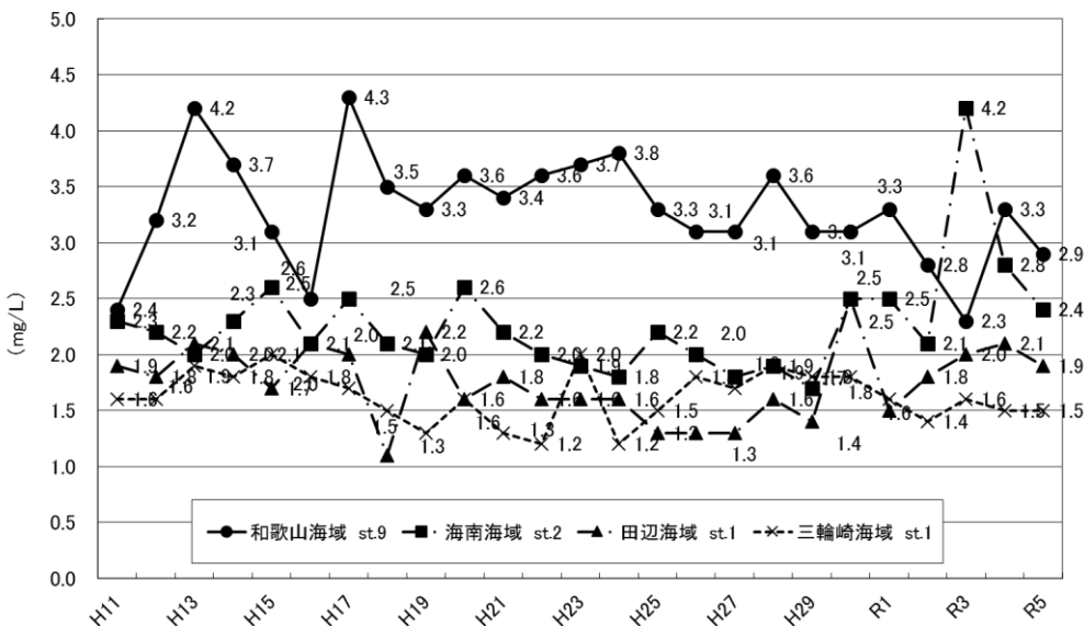
③ 主要海域の水質【COD】の推移 (75%値)
