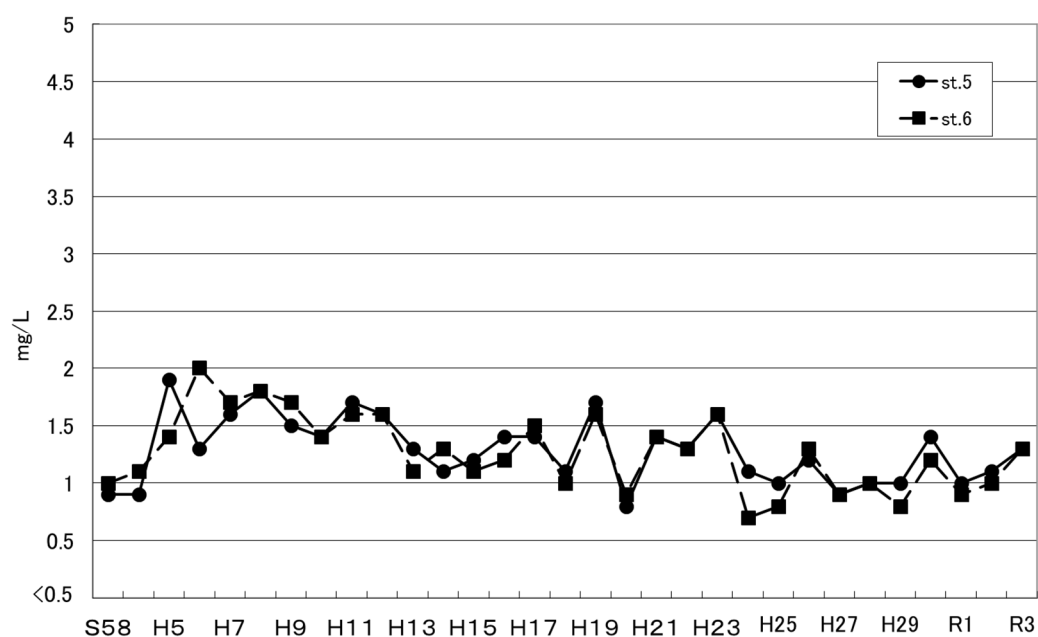
② 由良湾海域のCOD75%値の推移
