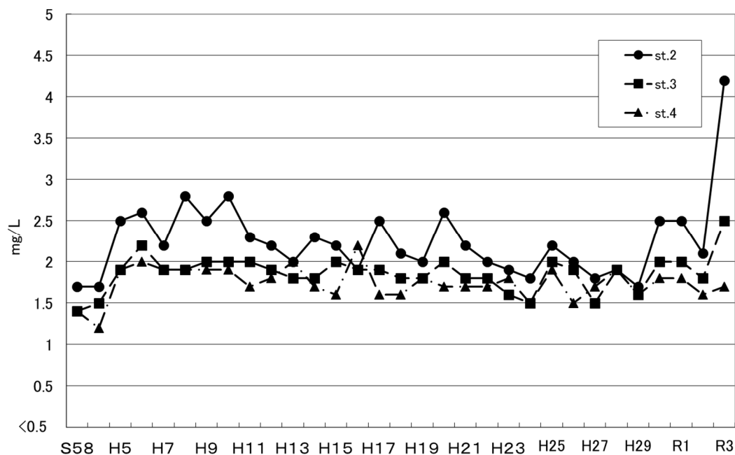
② 海南海域のCOD75%値の推移
