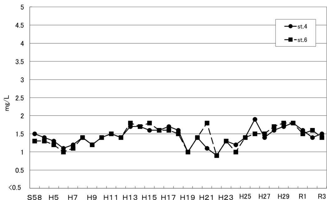
② 串本海域のCOD75%値の推移
