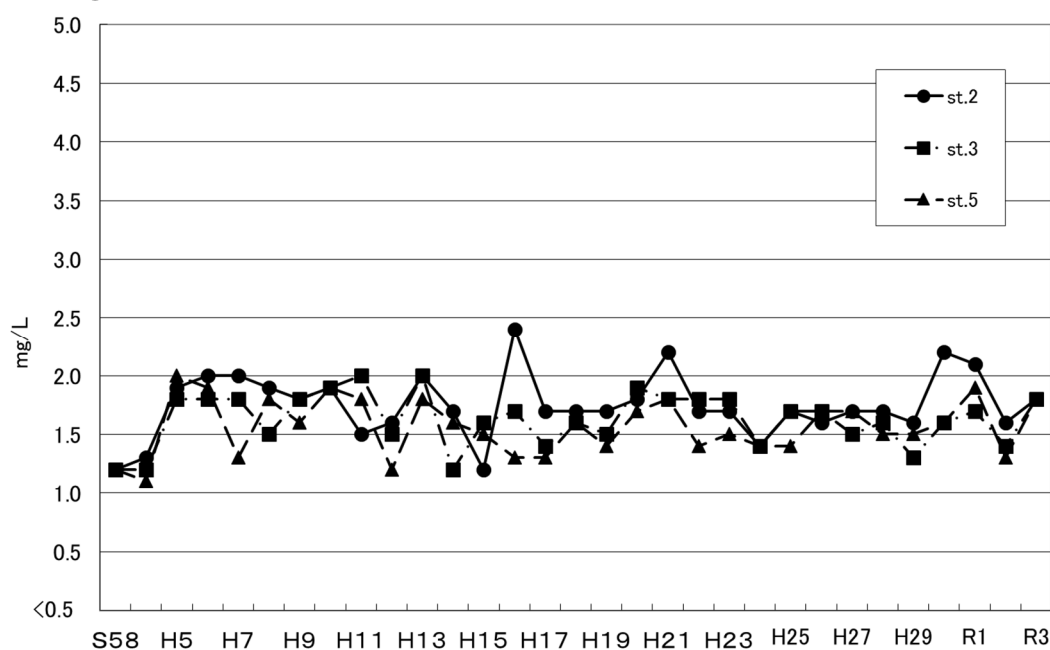
② 湯浅湾海域のCOD75%値の推移
