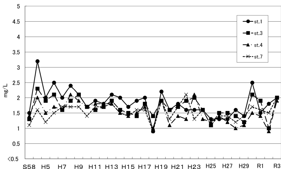
② 田辺湾海域のCOD75%値の推移
