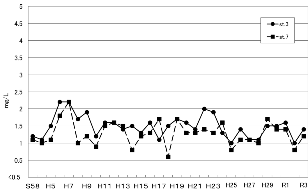
② 日高海域のCOD75%値の推移
