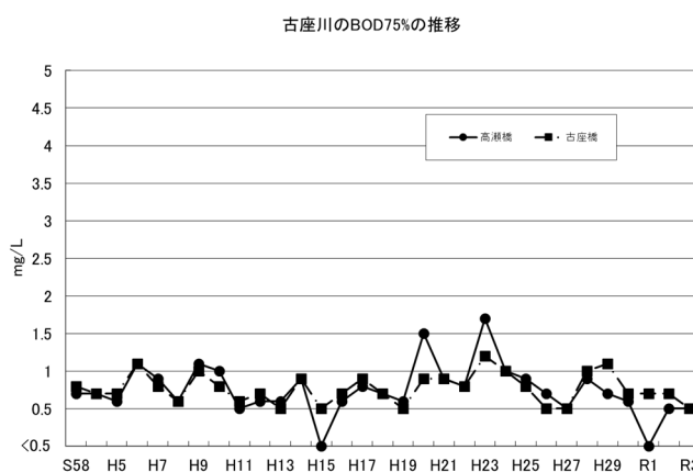
② 古座川のBOD75%値の推移
