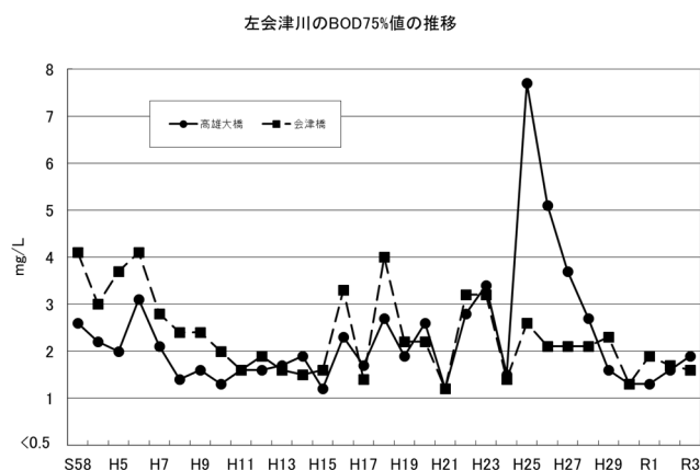
② 左会津川のBOD75%値の推移
