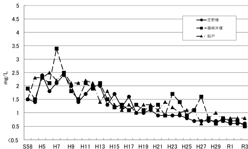
② 紀の川のBOD75%値の推移
