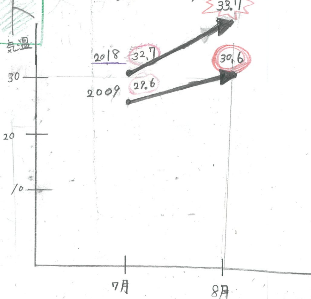
2009年と2018年の7、8月の平均気温
