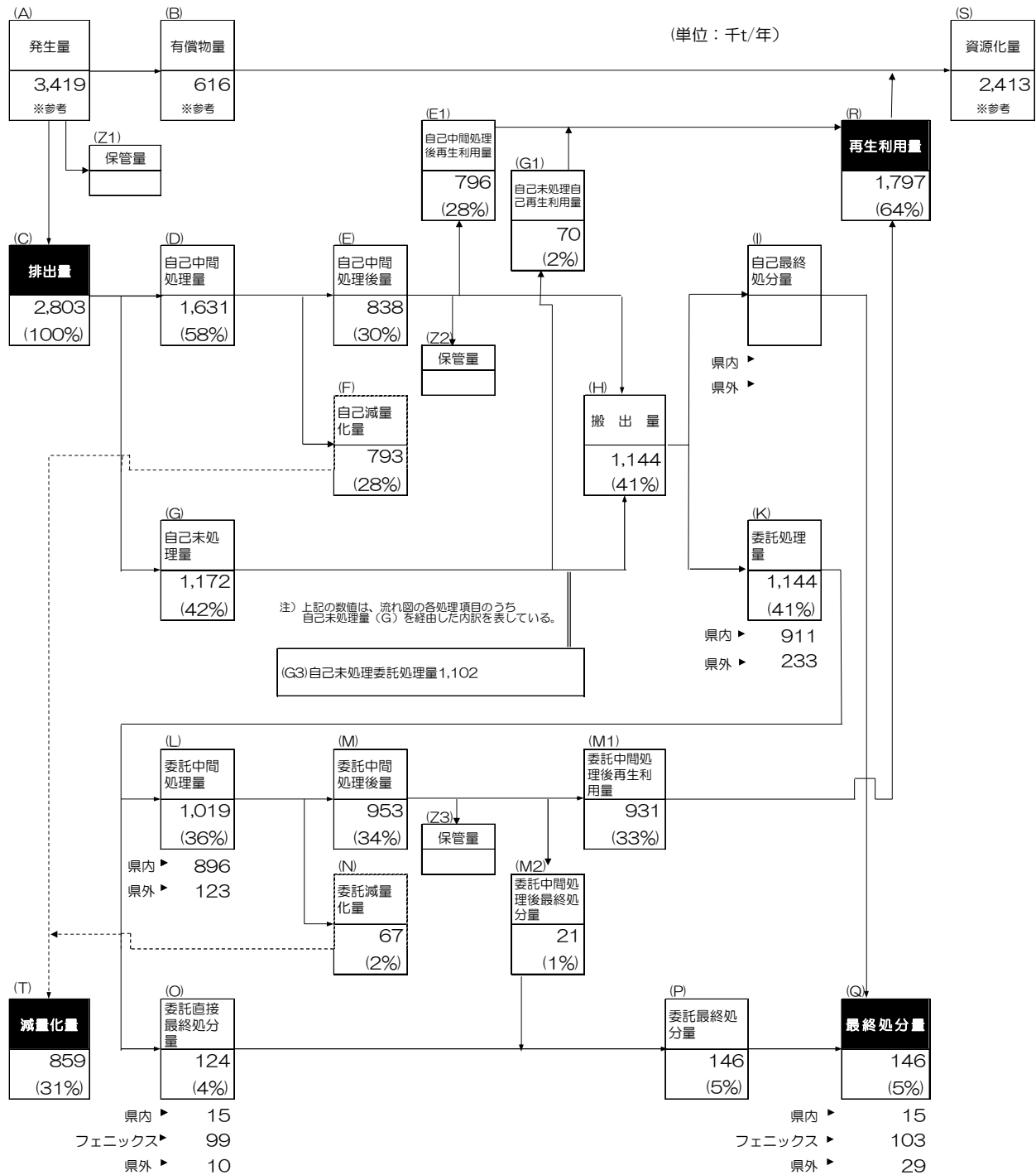
図表 3-1-8 産業廃棄物の排出及び処理フロー（2022（令和4）年度）
