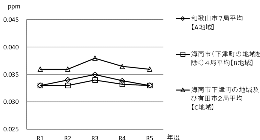
図表 4-1-10 光化学オキシダント濃度の 1 時間値の年平均値経年変化（発令地域別）
