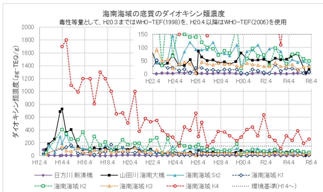
図表 4-5-9 底質調査結果の経年推移（2000（平成 12）年度～2023（令和 5）年度）
