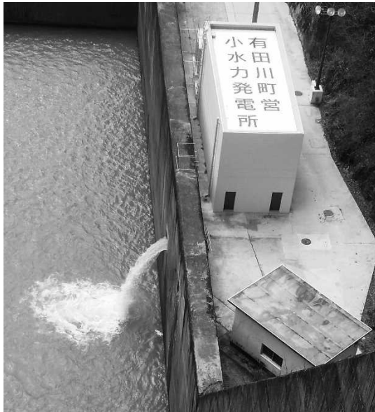
有田川町営二川小水力発電所
