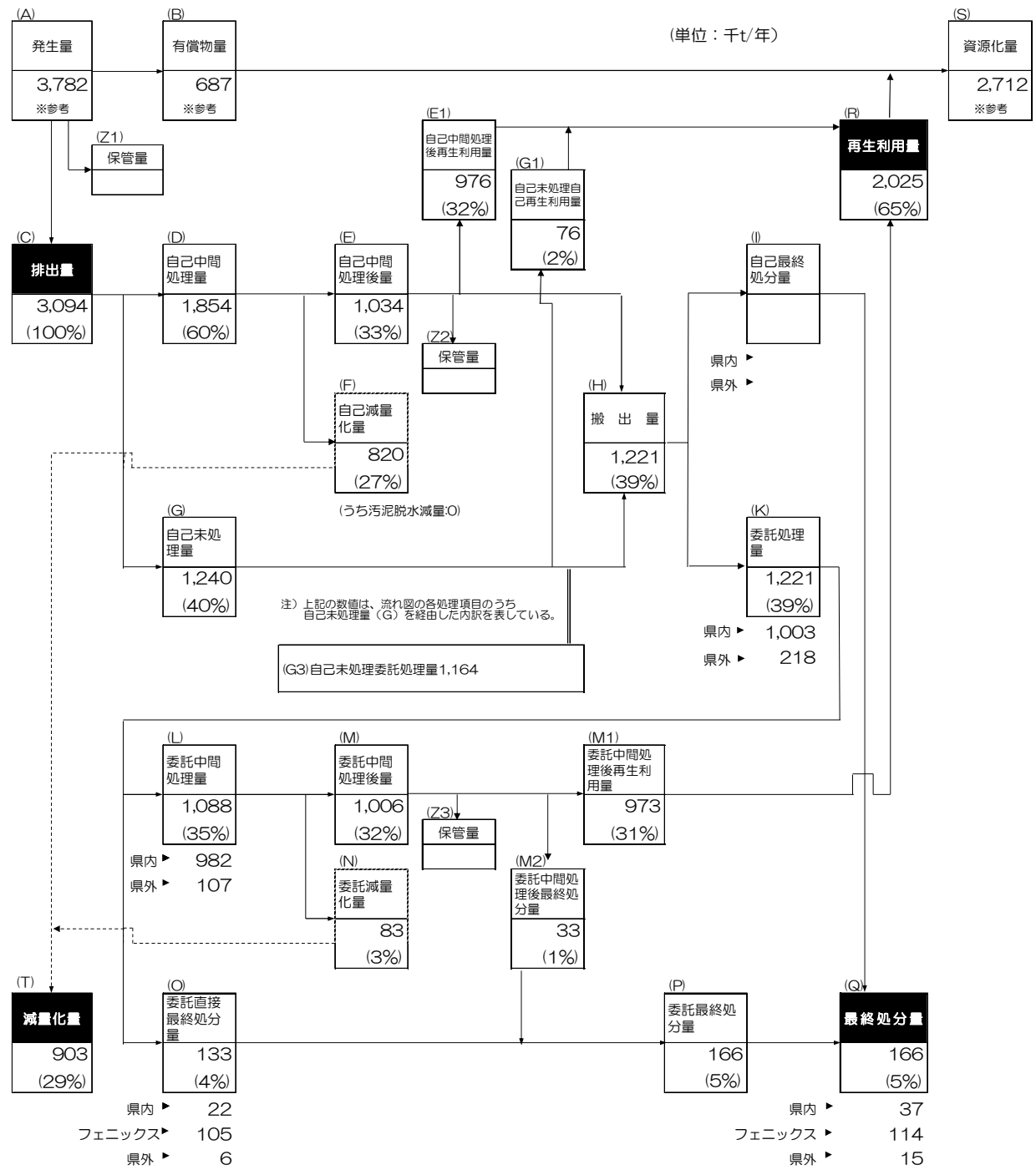
図表 3-1-8 産業廃棄物の排出及び処理フロー（令和2年度）
