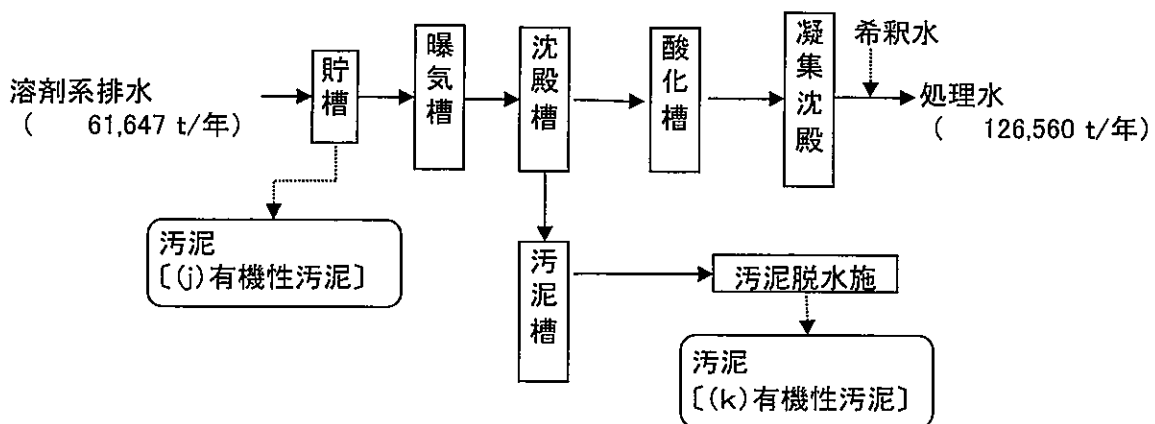
図5 排水処理フローシート[No6]
