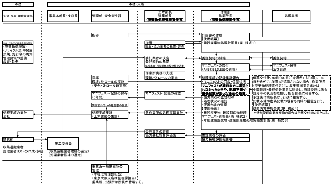
図ー1 産業廃棄物処理管理体系図
