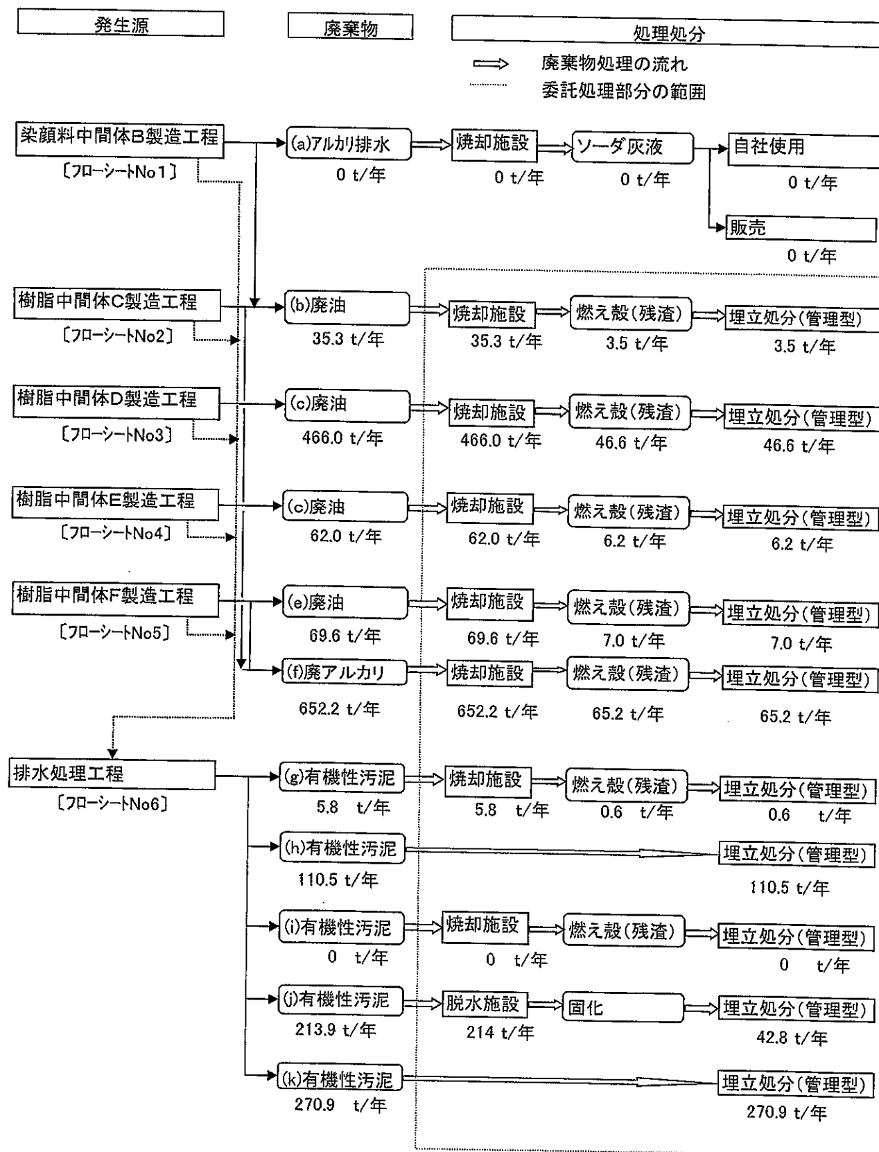
図6 廃棄物処理フローシート(現状)特管除く
