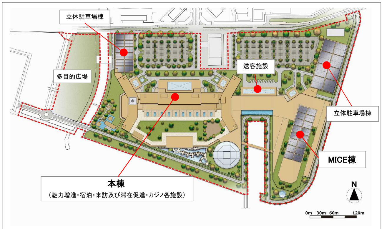
〈敷地配置図〉
