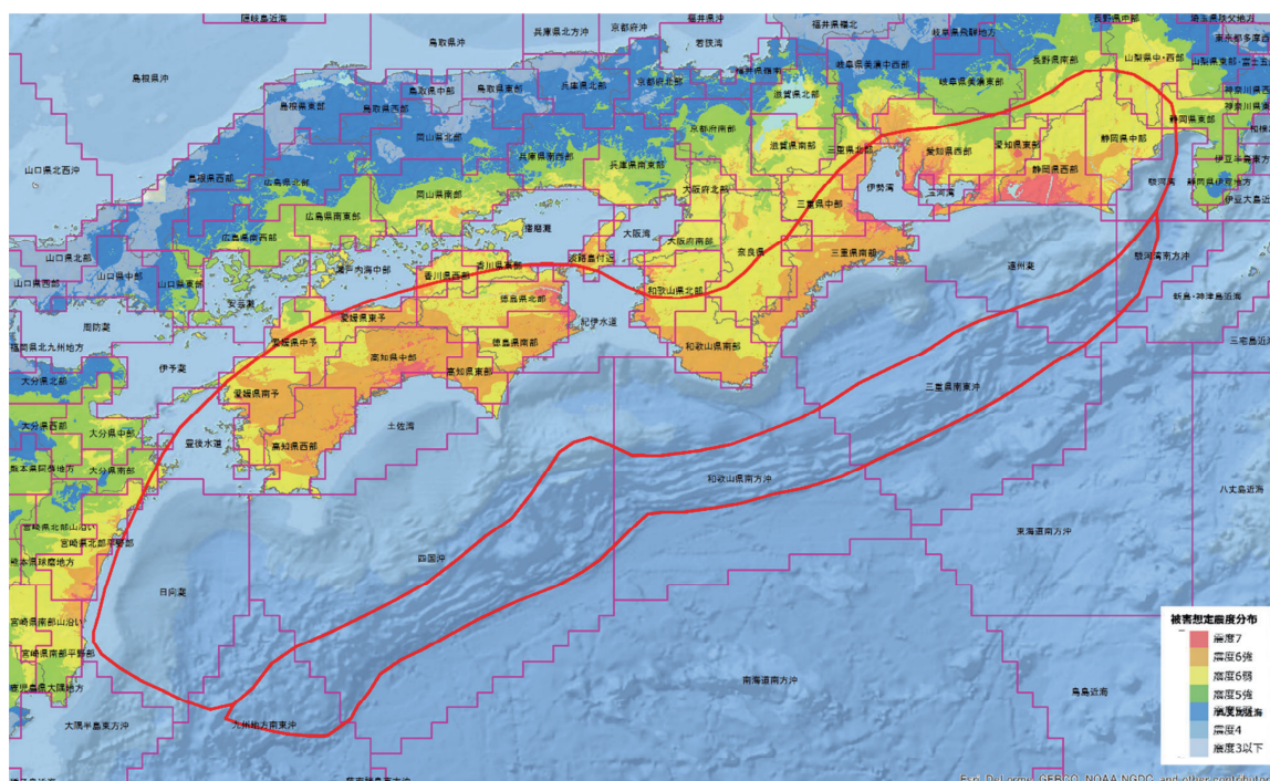
南海トラフ巨大地震の想定震源断層域と震央地名図
