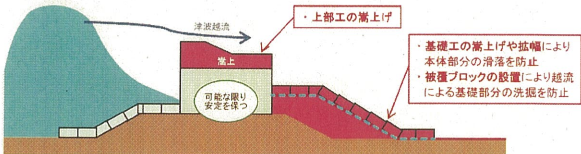
ねばり強い構造とすることで被害を押さえるための堤防強化について
