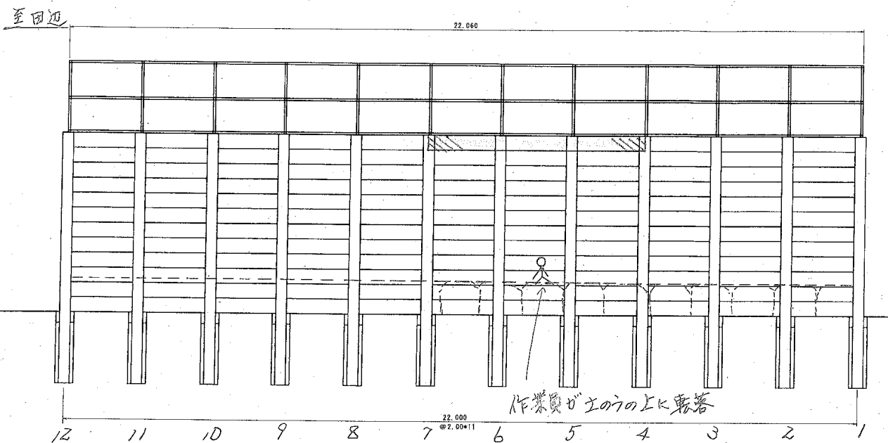
防護柵正面図 4-1/50
