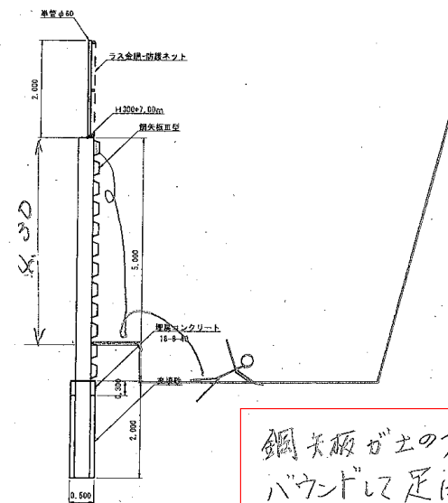
防護柵断面図 4-1/50
