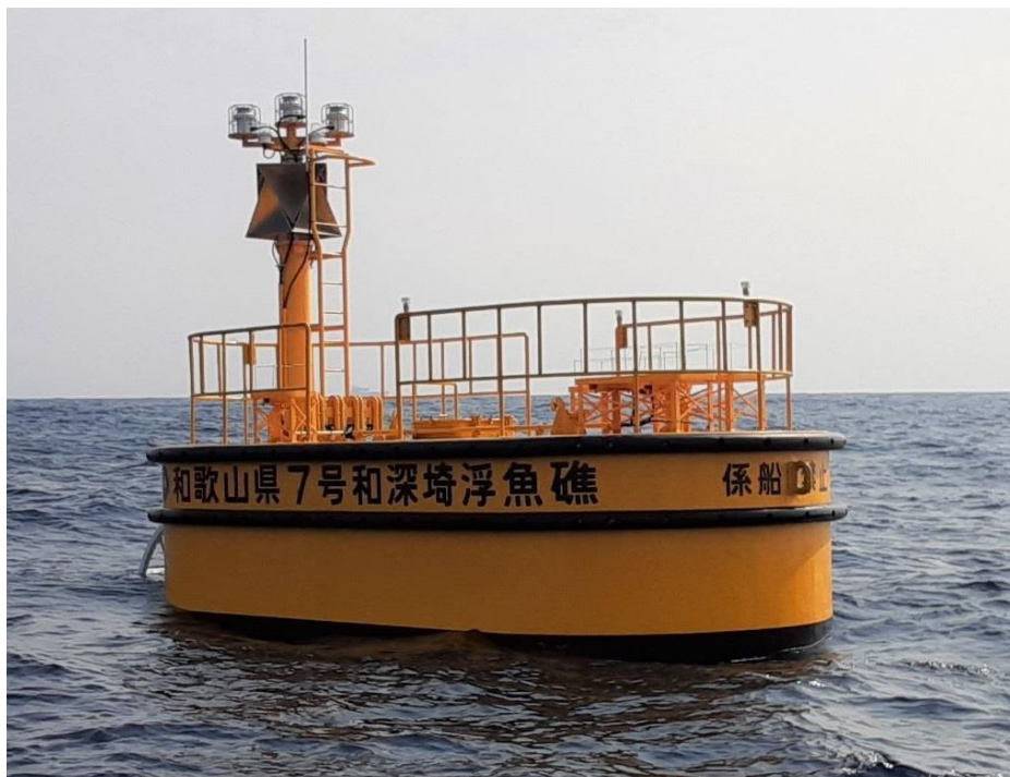
和歌山県7号和深崎浮魚礁 令和4年3月設置
