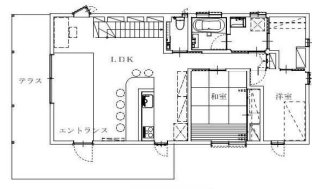
1階平面図
